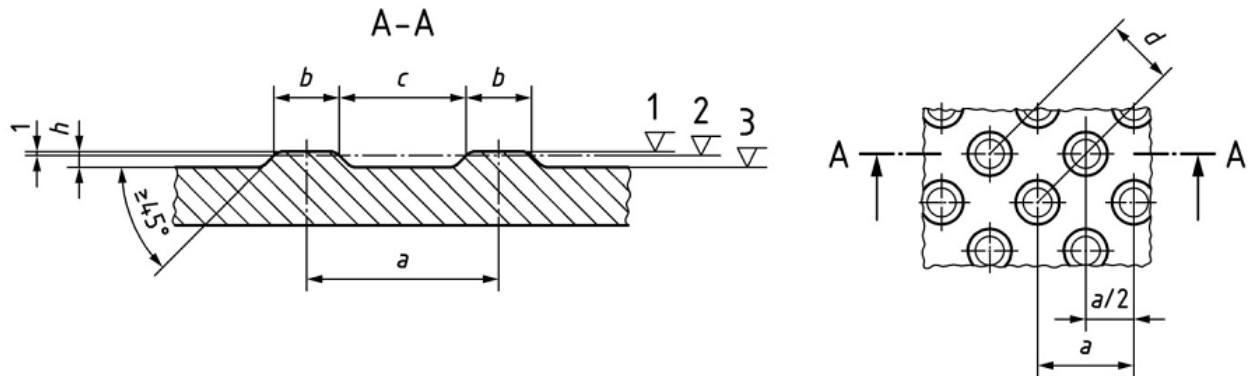
a = 58 \div 60 \text{mm} , b = 20 \div 22 \text{mm} , c = 37 \div 39 \text{mm} , d = 40 \div 42 \text{mm} , h = 4.5 \div 5 \text{mm} i (przy tolerancji 0.5mm) zawsze h > 4.5 \text{mm} Rys 2b. Wymiary wypustek płytki ostrzegawczej na podstawie normy DIN 32984
