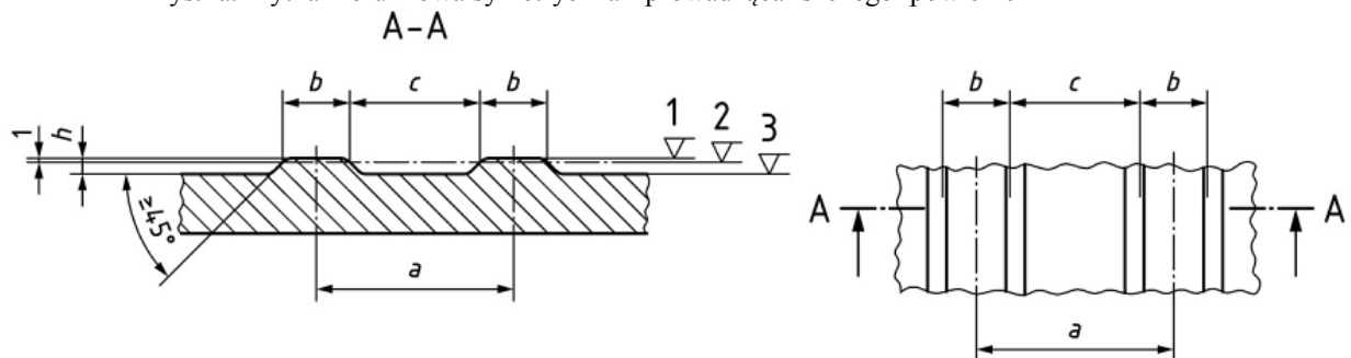
Rys. 1a. Płytki kierunkowa symetryczna - prowadząca- szczegól powierzchni
